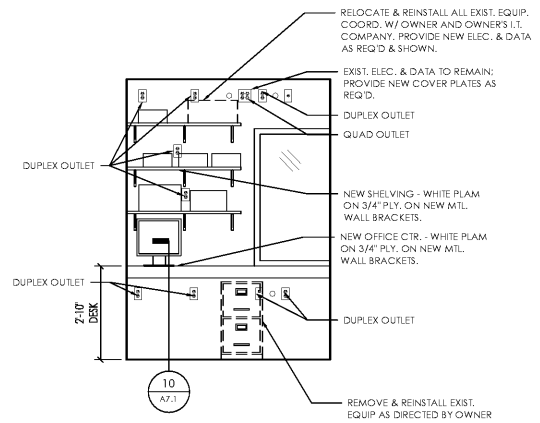
09 INT. ELEV @ OFFICE A7.1 SCALE: 3/8"= 1'-0"
