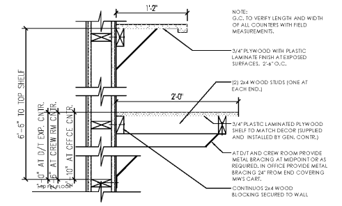
10 MILLWORK DTL A7.1 SCALE: 1"= 1'-0"
