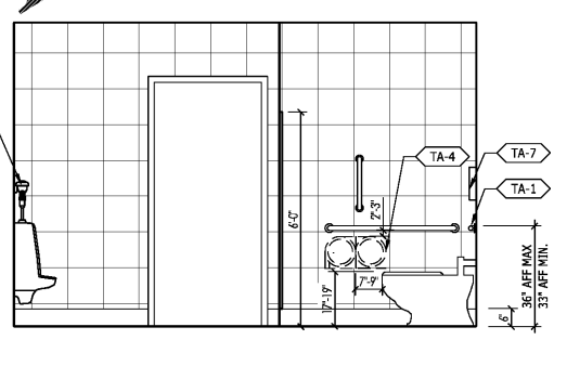
02 INT. ELEV @ MEN'S A7.1 SCALE: 3/8"= 1'-0"
