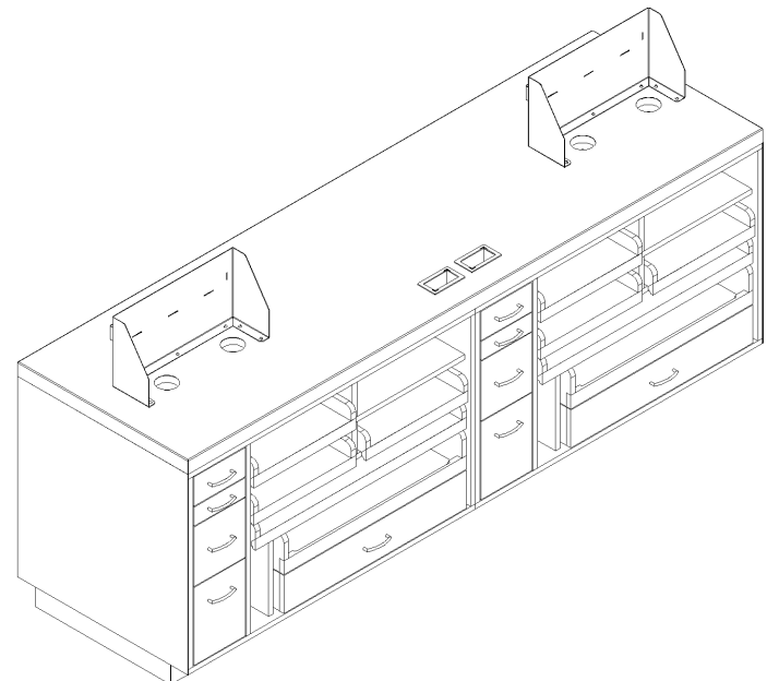
C REAR CASHWRAP ISOMETRIC N.T.S.
