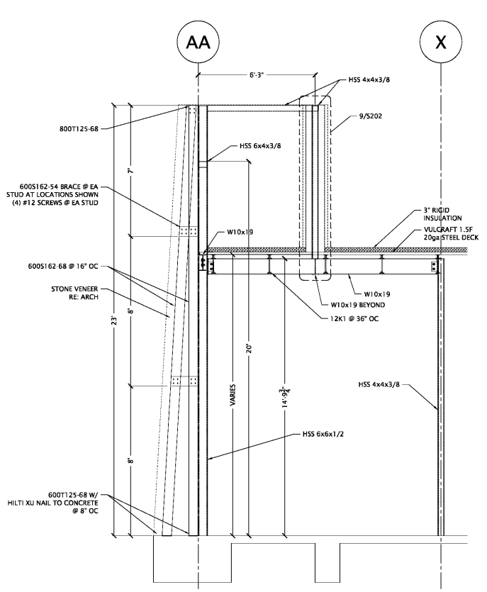
1 SECTION SCALE: 3/8" = 1'-0"
