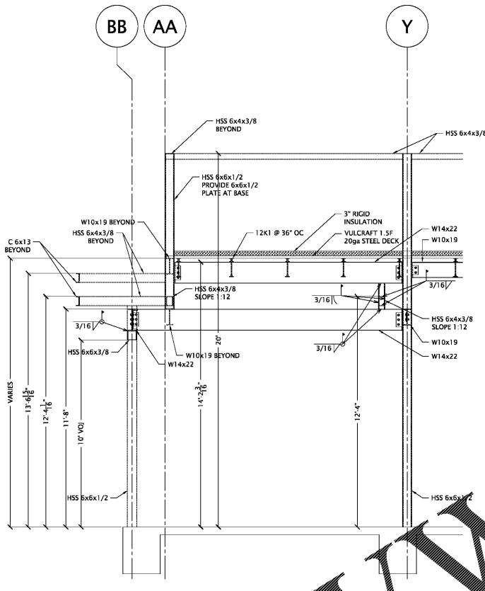
2 SECTION SCALE: 3/8" = 1'-0"
