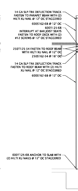
7 ELEVATION (CFS) SCALE: 3/8" = 1'-0"
