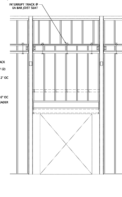
6 SECTION (CFS) SCALE: 3/8" = 1'-0"
