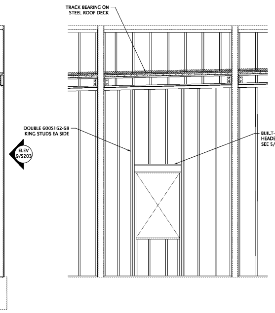
7 ELEVATION (CFS) SCALE: 3/8" = 1'-0"
