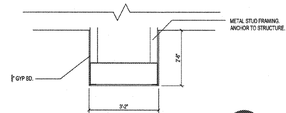
1 SOFFIT DETAIL AI-08 SCALE: 1/2" = 1'-0"
