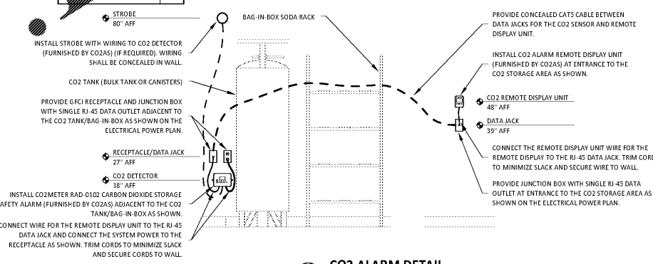
12 E300 CO2 ALARM DETAIL N.T.S.
