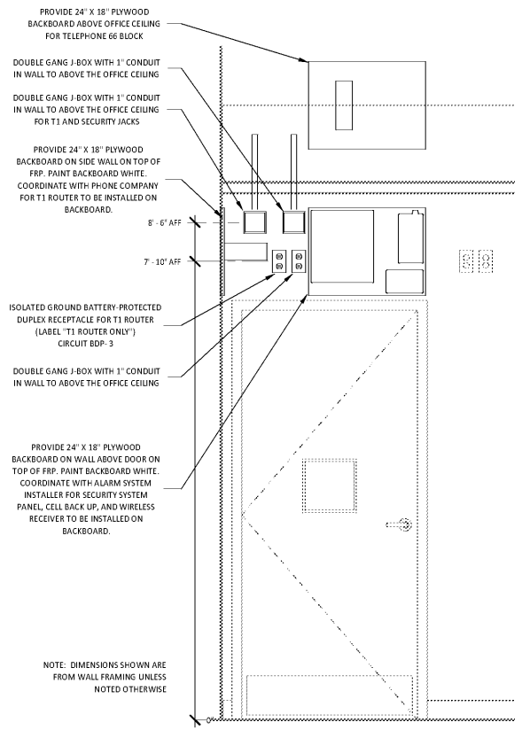
10 E300 OFFICE DOOR ELECTRICAL ELEVATION N.T.S.
