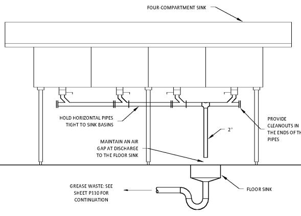
4 WARE-WASHING SINK DETAIL P300 N.T.S.
