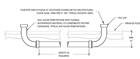
7 SODA CONDUIT DETAIL P300 N.T.S.
