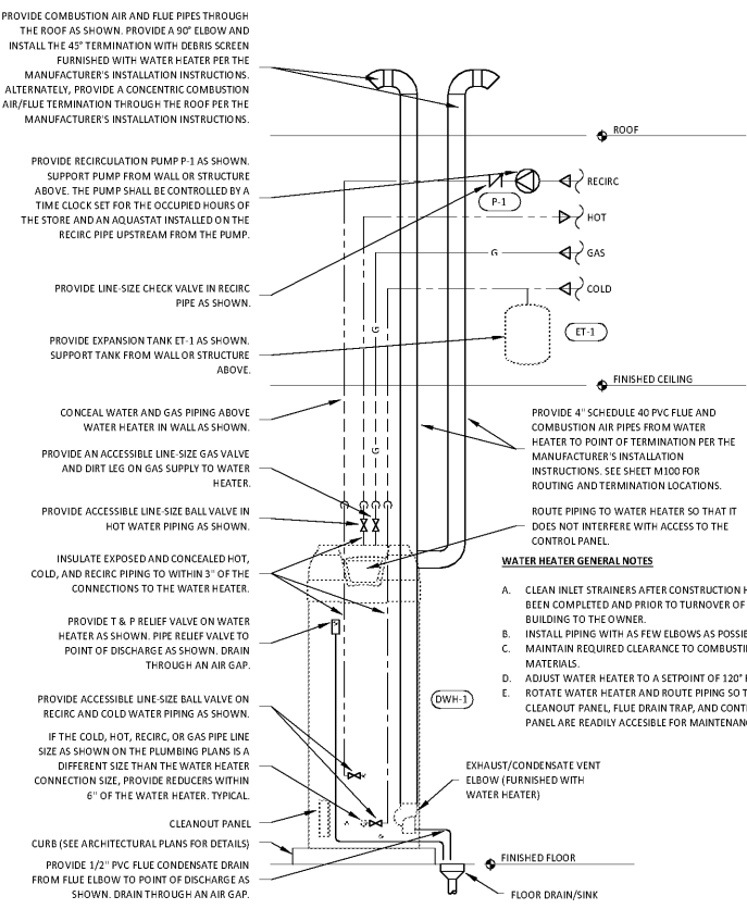
1 WATER HEATER DETAIL P300 N.T.S.
