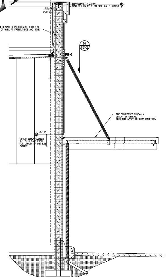
2 SECTION FS-3 SCALE: 1/2"=1'-0"
