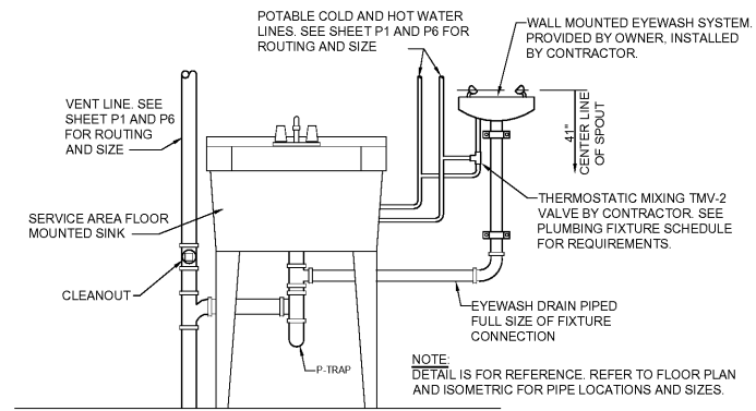
5 EYEWASH PIPING DETAIL P5 SCALE: N.T.S.
