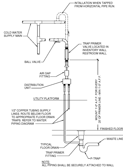
2 TRAP PRIMER DETAIL (TP-1) P5 SCALE: N.T.S.
