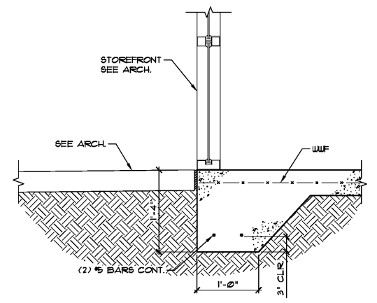
12 SECTION SCALE: 1" = 1'-0"
