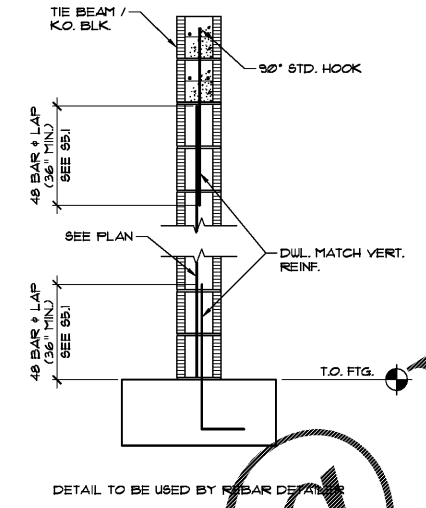
6 SECTION SCALE: 3/4" = 1'-0"
