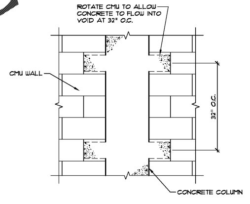
8 SECTION SCALE: 3/4" = 1'-0"
