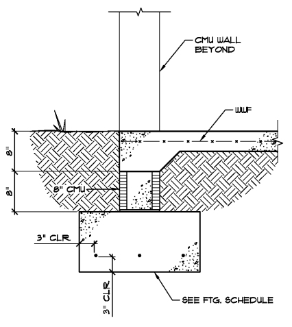
2 SECTION SCALE: 1" = 1'-0"
