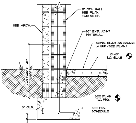
5 SECTION SCALE: 1" = 1'-0"
