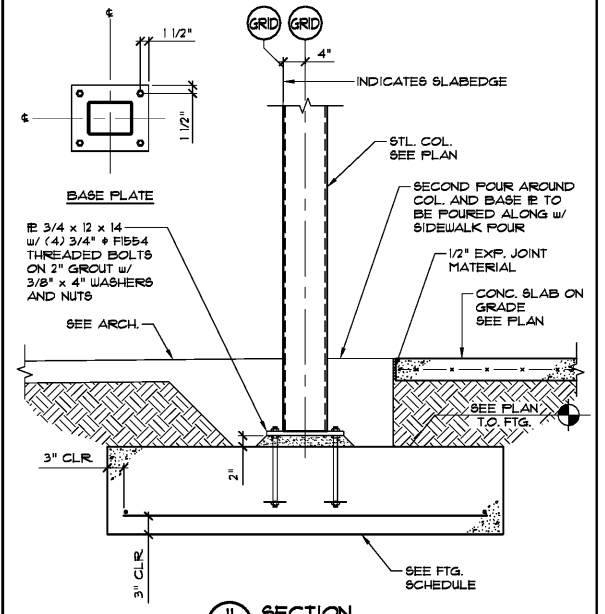
11 SECTION SCALE: 3/4" = 1'-0"
