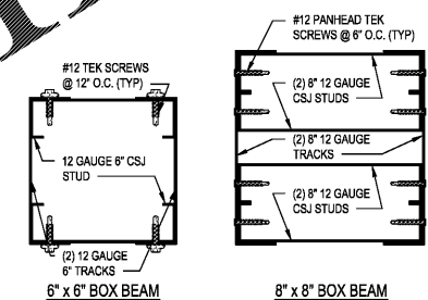
BOX BEAM DETAILS SCALE: 3"=1'-0"
