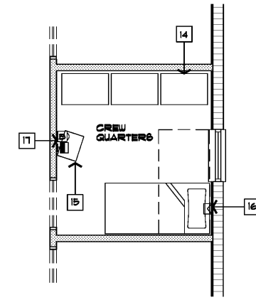
(D) PARTIAL ENLARGED FLOOR PLAN SCALE 1/4" = 1'-0"
