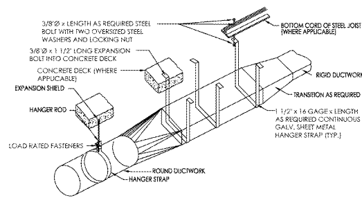
TYPICAL DUCT TRAPPING DETAIL SCALE: N.T.S.
