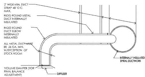
ROUND DUCT DETAIL SCALE: N.T.S.
