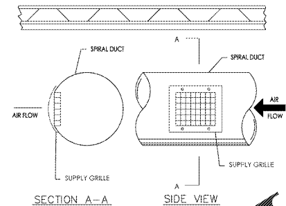
DUCT MOUNTING DETAIL SCALE: N.T.S.
