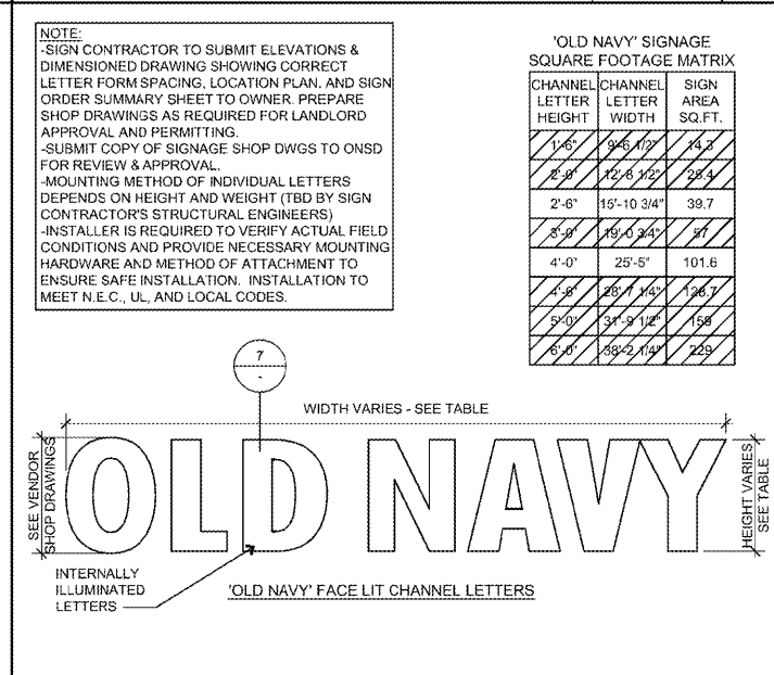
CHANNEL LETTER SIGNAGE - FACE ILLUMINATED SCALE: N.T.S. 1
