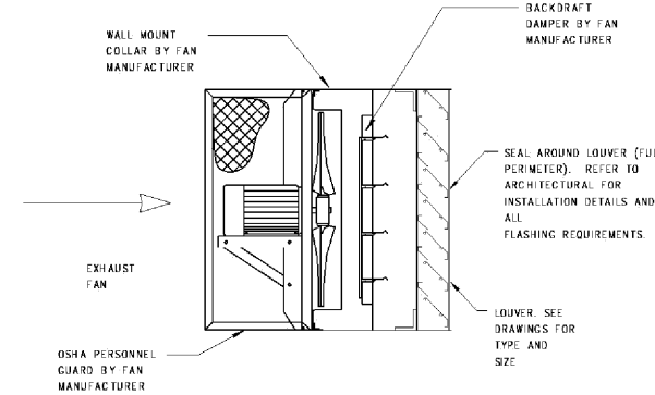
SIDEWALL FAN DETAIL
